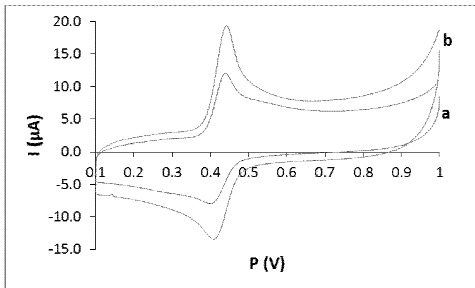
Figure 1: Voltammogrammes cycliques de (a) SPCE et (b) Al-CuSe-NPs / ECS dans 0,1 mM de la dopamine et H 3 PO 4 0,1 M.
