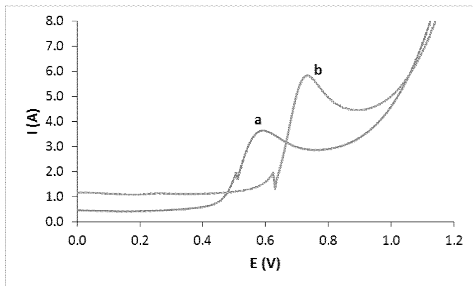
Figure 2: Voltammogrammes de balayage linéaire de L-tyrosine à 30 µM dans un tampon H 3 PO 4 0,1 M à pH = 2,0, vitesse de balayage de 50 mV / s de (a) ECS et (b) Al-CuSe-NPs / ECS.
