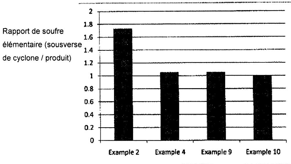
Figure 4 - Rapports de soufre élémentaire pour la sousverse de cyclone de séchoir pour différents additifs tensioactifs
