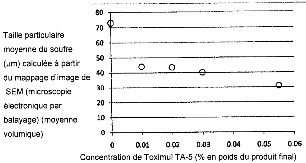
Figure 3 - Taille particulaire moyenne du soufre dans les granulés d'engrais, pour différentes concentrations de Toximul TA-5
