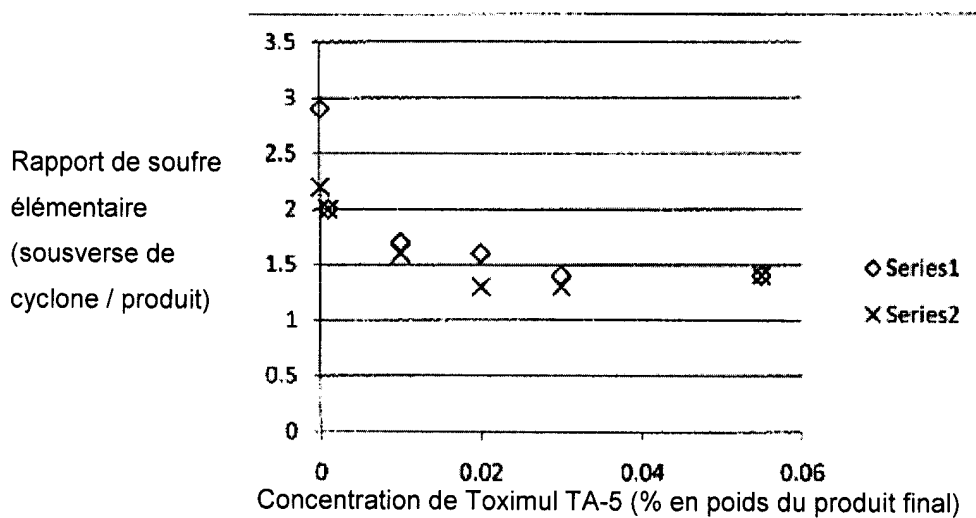
Figure 2 - Rapports de soufre total pour les surverses de cyclone de séchoir (série 1) et de poussière fugitive (série 2) pour différentes concentrations de Toximul TA-5
